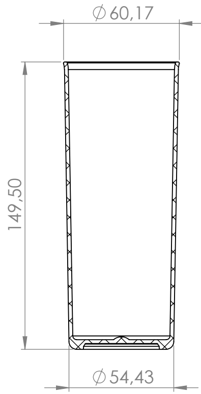
SEÇÃO A-A
